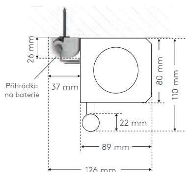
Montáž na strop D
