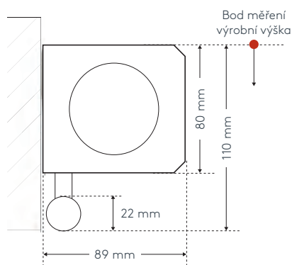
Montáž na stěnu W
