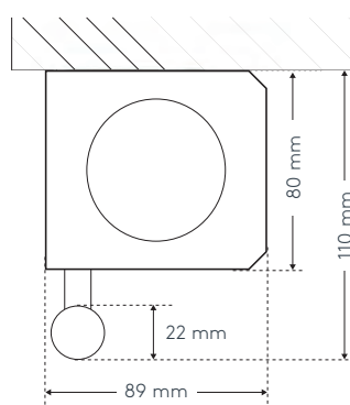
Montáž na strop D
