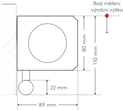
Montáž na stěnu W
