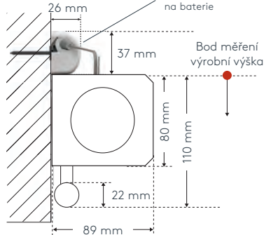
Montáž na stěnu W
