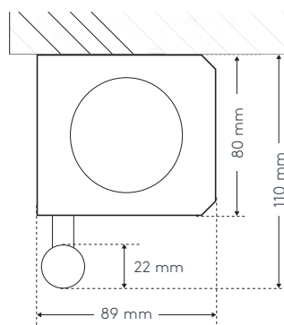
Montáž na strop D
