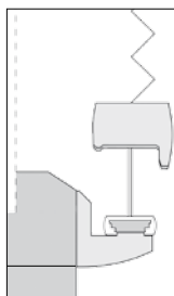
Řez okenním rámem s plastovým držákem a dolním profilem
