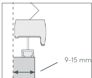
Řez zasklívací lištou s upínací patkou a dolním profilem
