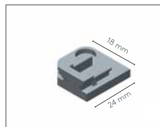
Upínací patka kulatá Č. art. 29.7929
