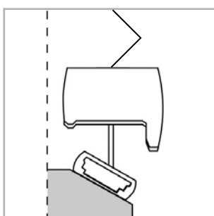
Upravený dolní profil pro šikmou zasklívací lištu, navíc zakrývající upínací patky
