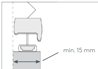
Řez zasklívací lištou s upínací patkou a dolním profilem
